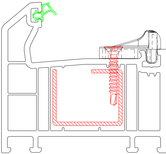
10825 - İspanyolet Karşılık 13 destek sacına vidalanmaktadır.
